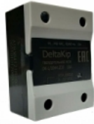
Однофазное твердотельное реле DK1-4025.DD3
